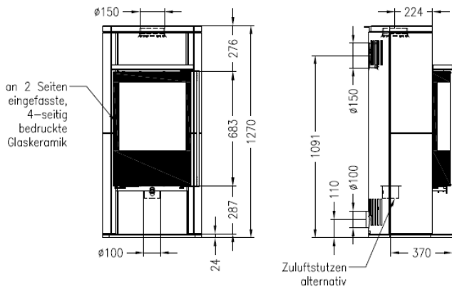
Vorderansicht M~1:20
